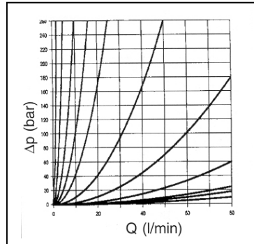
Szabályozott térfogatáram
