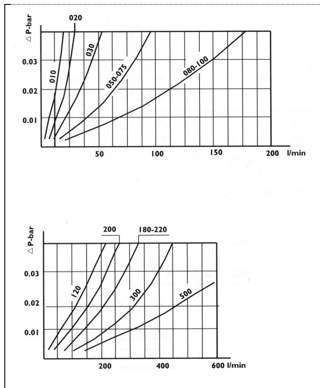
Térfogatáram – nyomásesés, olaj: 36 cSt, 40 °C, szűrés: 90 µm
