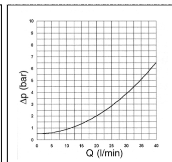
Szabad átfolyás a visszacsapón keresztül
