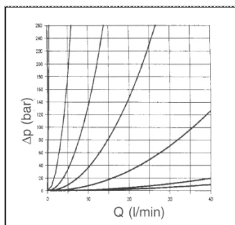
Szabályozott térfogatáram
