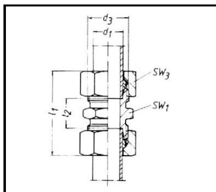
Beépítési méretek
